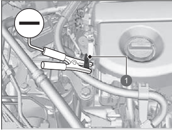
1 Stud Bolt
